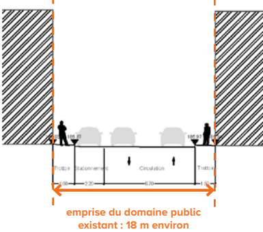
Coupe type existant - rue Émile Zola ouest
