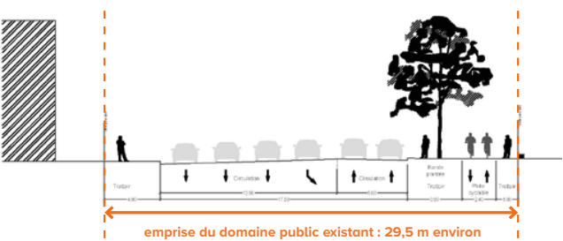
Coupe type existant - avenue Tony Garnier
