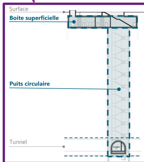
Schéma de principe d'un puits
